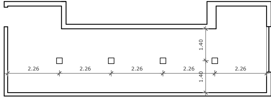
2 PLANTA BAIXA - ALMOXAFIRADO ILUMINAÇÃO ESCALA: 1:100
